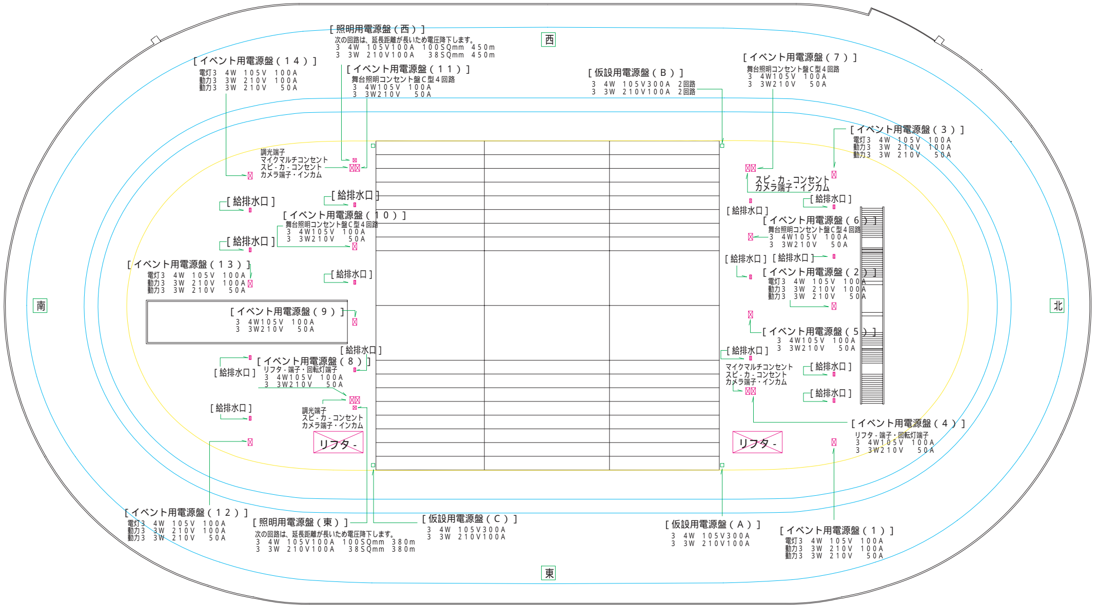
グリーンドーム前橋 設備平面図 ハンドホール配置 1/400 2000年10月1日現在
